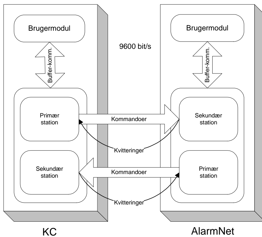
Fig. B.2. ALC/FD - primær og sekundær station
